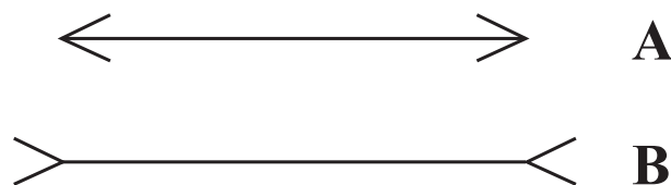
Ryc. 1. Iluzja Müller-Lyere.
